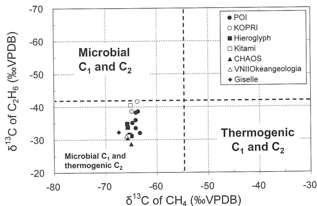
図 4 ハイドレート解離ガスのメタンおよびエタンの \delta^{13}\text{C} の関係。
